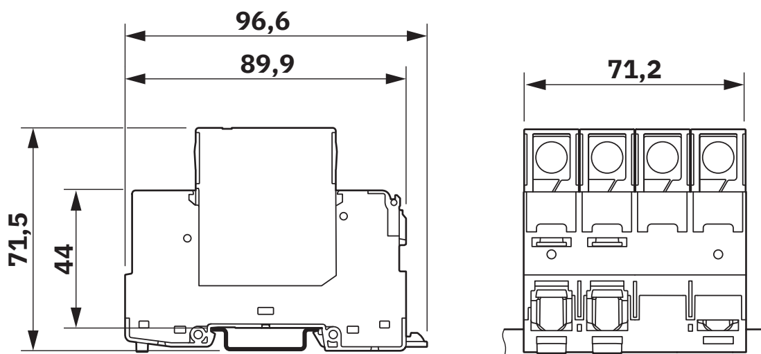
Méretrajz
